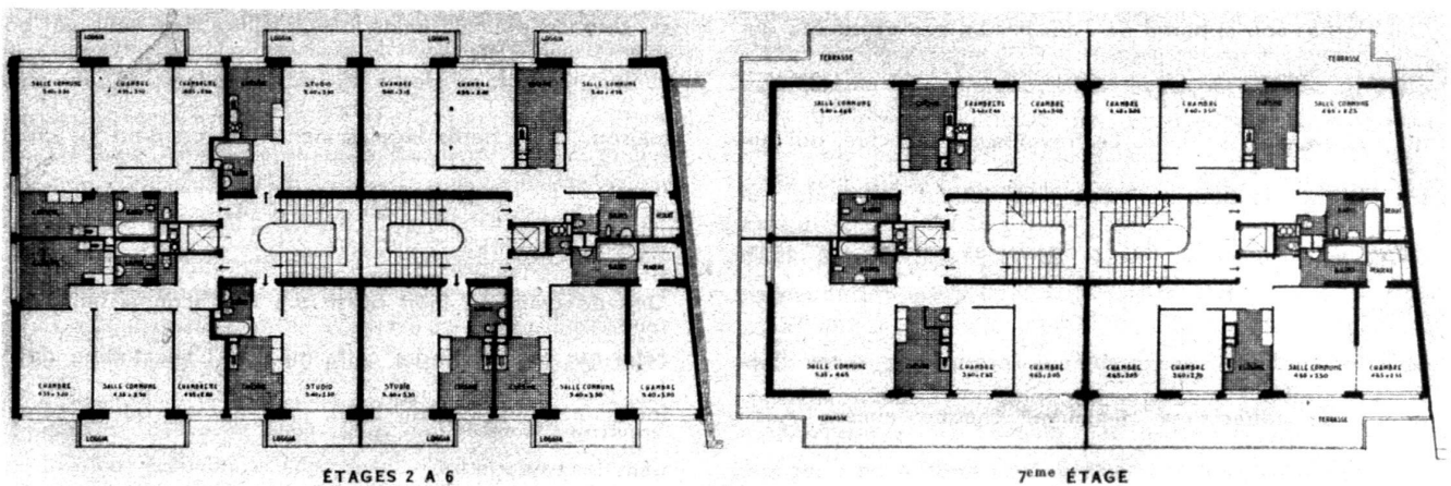
Plan des étages.
