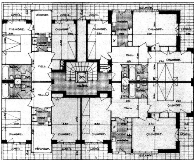
Plan des étages.
