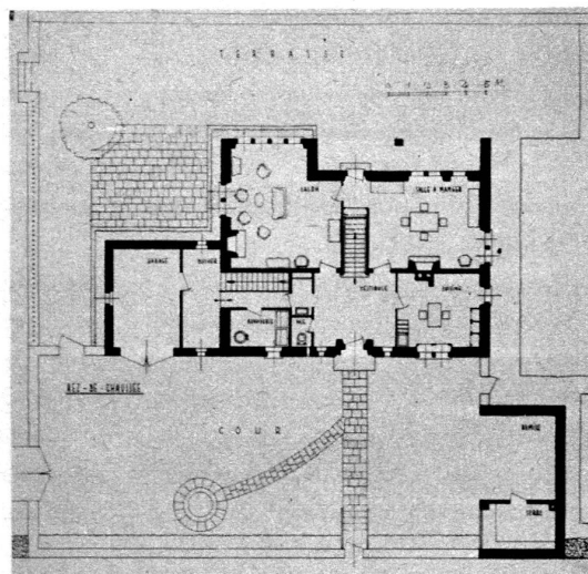
Maison à Cologny, rez-de-chaussée
