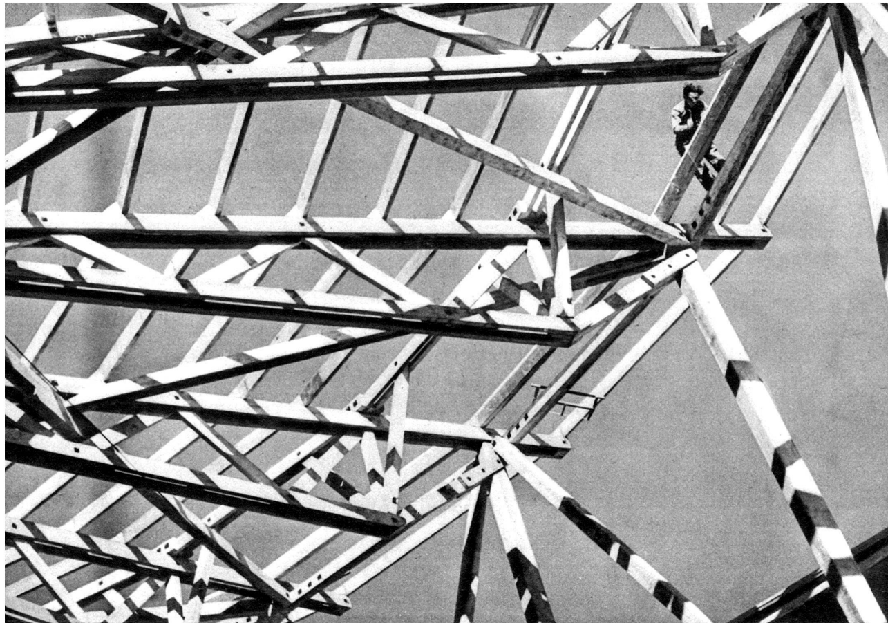
La charpente du Pavillon des transports est aujourd'hui terminée et couverte. Cette photo a permis d'en fixer l'aspect aérien qui intéressera surtout nos constructeurs.
