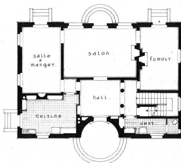
Rez-de-chaussée. Ech. : 1/200.
