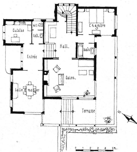
Rez-de-chaussée. Ech. : 1/300.
