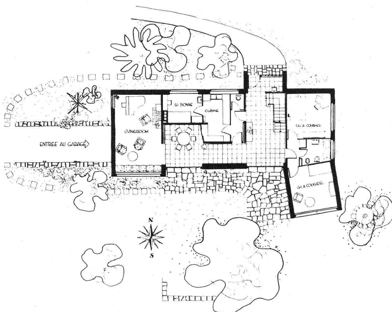
Rez-de-chaussée. Ech. : 1/300.
