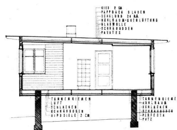
Coupe 1 : 200.
