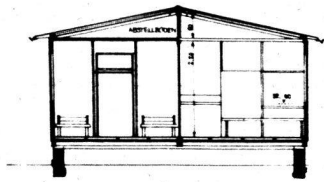
QUERSCHNITT
