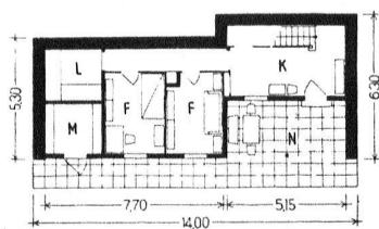
Sous-sol.
