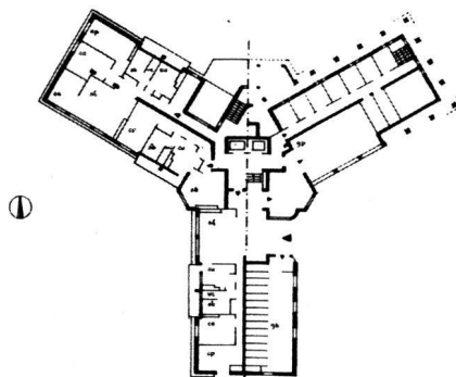
b plan du rez-de-chaussée et d'étage courant
