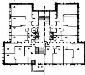
b 1/2 plan rez. et étage courant
