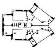
a variante plan d'appartement
