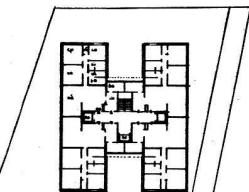
a plan d'étage courant
