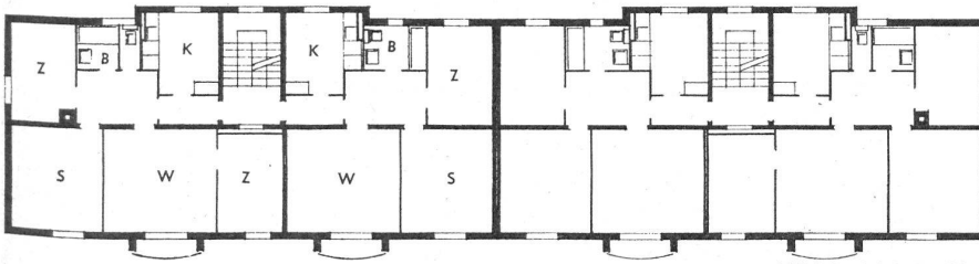
Plan 1 : 300.
