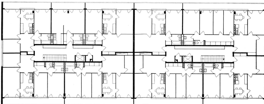
Plan, échelle 1 : 300.
