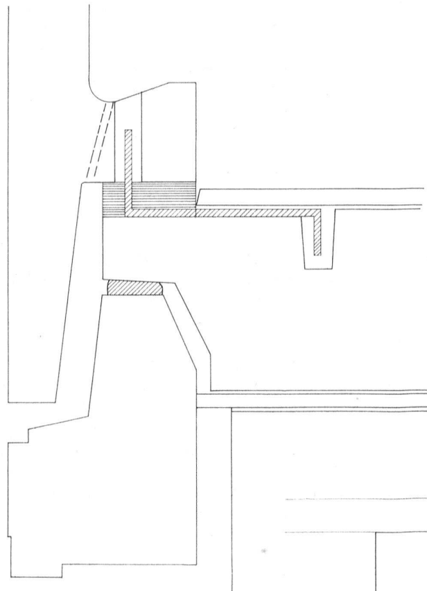
Coupe verticale
