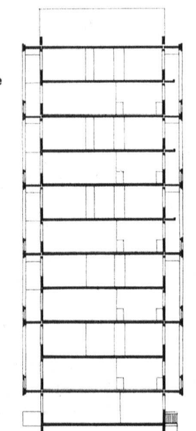
Coupe, échelle 1:400
