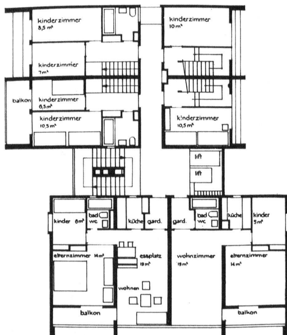
Plan d'étage, Berne-Bümpliz.
