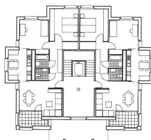
Plan type, rez-supérieur, 1 er étage.
