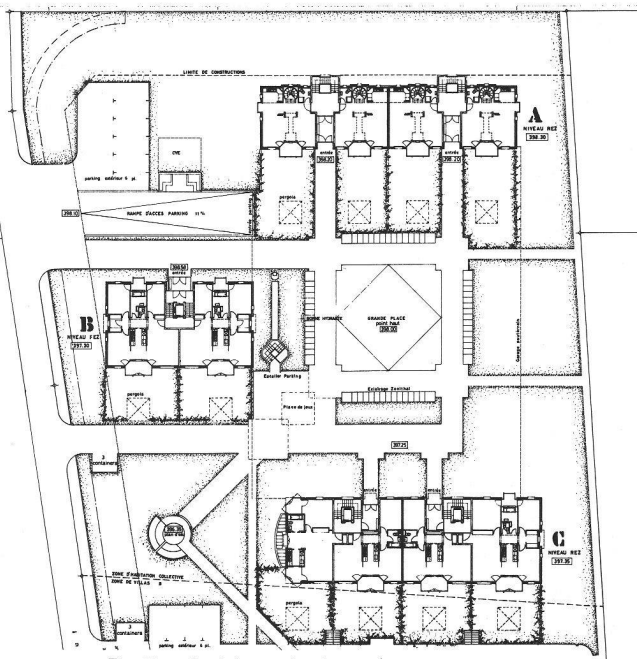
Fig. 7 — Projet: rez-de-chaussée.
