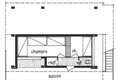
REZ INFÉRIEUR
