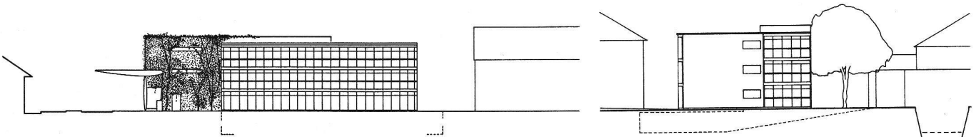
FACADE SUD-OUEST
