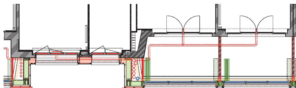
0 1 2 5 PLAN TYPE DES LOGGIAS
