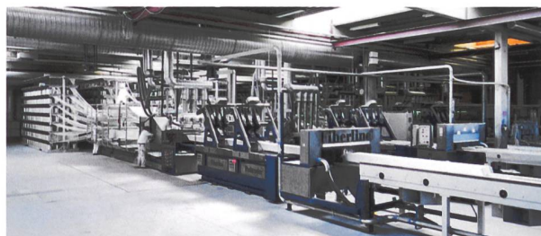
Halle de fabrication de barres en matériaux composites. Pultrusion 1/ DR
