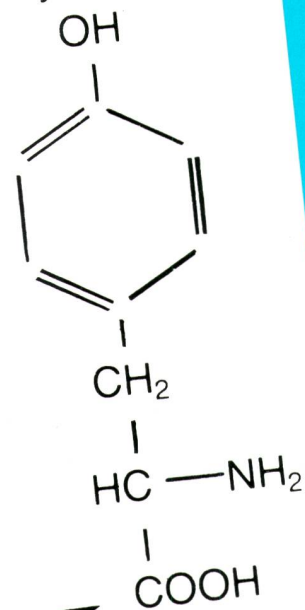
Tyrosin
