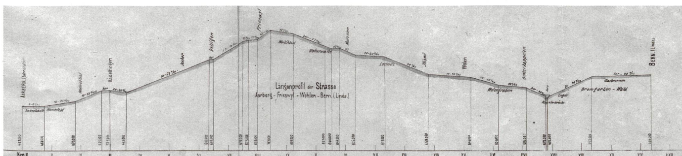
Längenprofil der Strasse von Aarberg über Wohlen nach Bern/Linde, mit der Kappelenbrücke zwischen km XVII und XVIII (StAB BB 10.3.134_44 A1 13 a/b)
