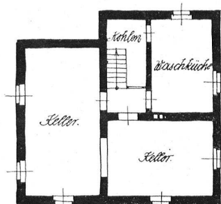
Grundrisse 1 : 250
