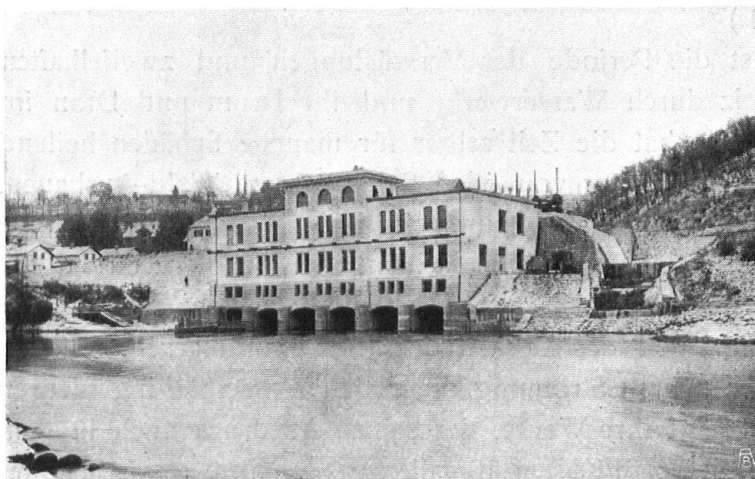
Abb. 8. Gegenbeispiel . Turbinenhaus des Wasserwerks Felsenau bei Bern. Nüchterner, unerfreulicher Bau. — Fig. 8. Mauvais exemple . Bâtiment des turbines des installations hydrauliques de Felsenau, près Berne. Construction banale.
