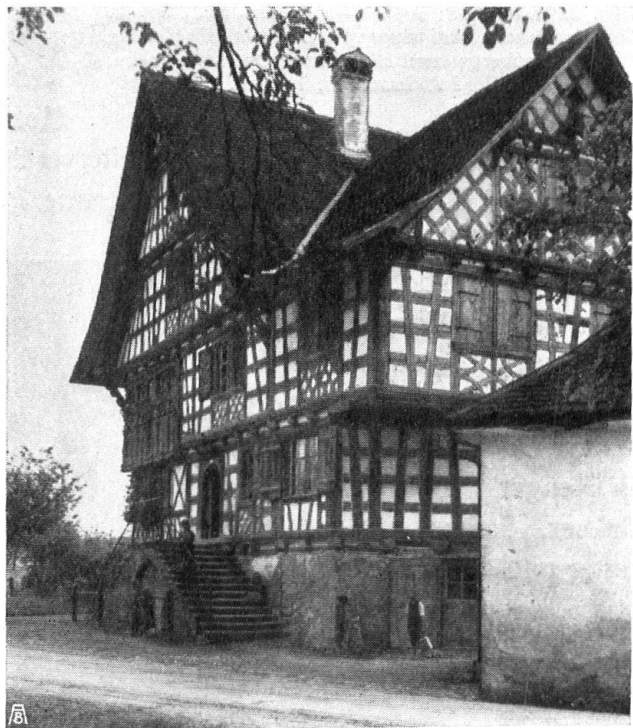
Abb. 1. Riegelhaus bei Oberaach im Thurgau. Teils Holzbau, teils Fachwerk in schöner Zeichnung. Aufnahme von Hausmann in Heiden. — Fig. 1. Maison en colombage, près Oberaach, en Thurgovie. Construction partie en bois, partie en colombage (pan de bois) et de formes agréables. Cliché Hausmann, à Heiden.
