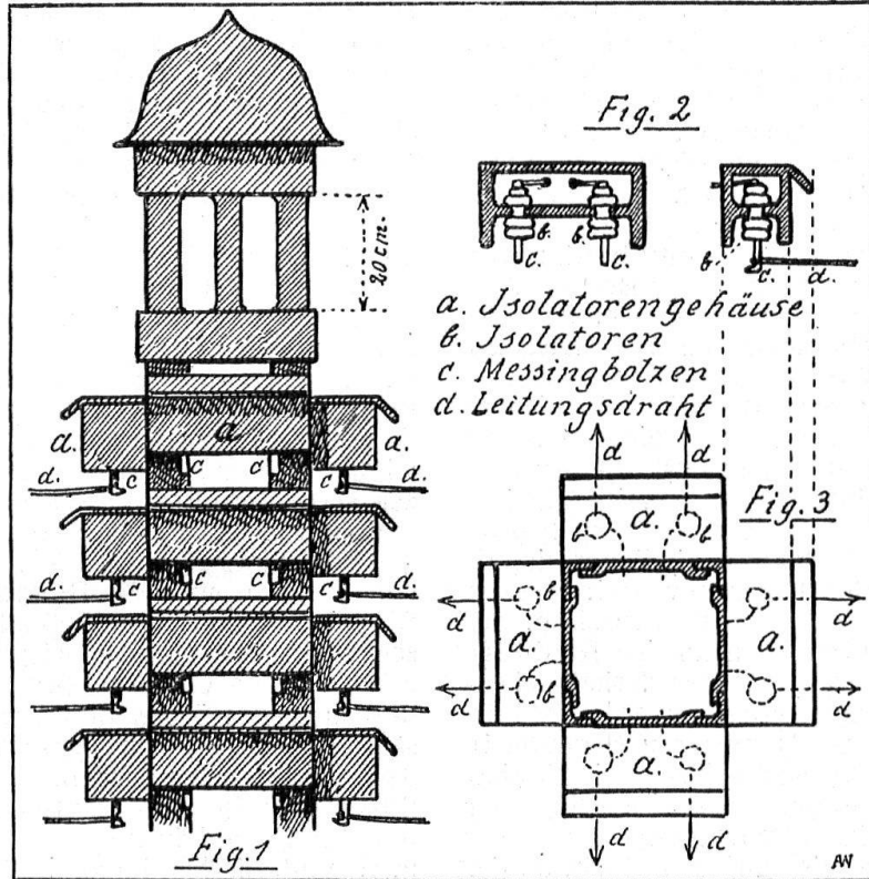
Abb. 18. Telephonmasten-Wettbewerb. Projekt Helbock. Fig. 1. Ansicht des Verteilungskorbes. Fig. 2. Senkrechter Schnitt durch die Isolatorgehäuse. Fig. 3. Wagerechter Schnitt durch die Kabelsäule über den Isolatorgehäusen.
