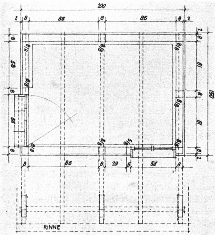
Abb. 5. Prämiierter Entwurf „Gäli Rüebe“. Grundriss. — Fig. 5. Projet primé „Gäli Rüebe“. Plan.
