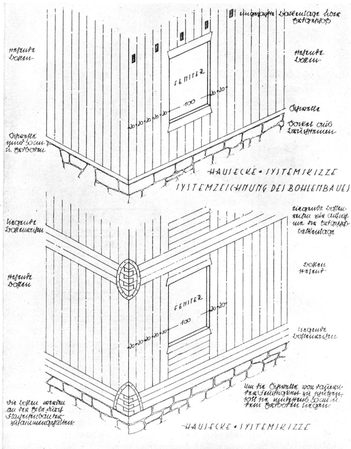
Wandsysteme und Eckausbildung im Bau aus stehenden Bohlen. Aus dem Buche von Stolper: «Bauen in Holz». — Détails de la construction des parois et des angles, d'après l'ouvrage très recommandable «Bauen in Holz».
