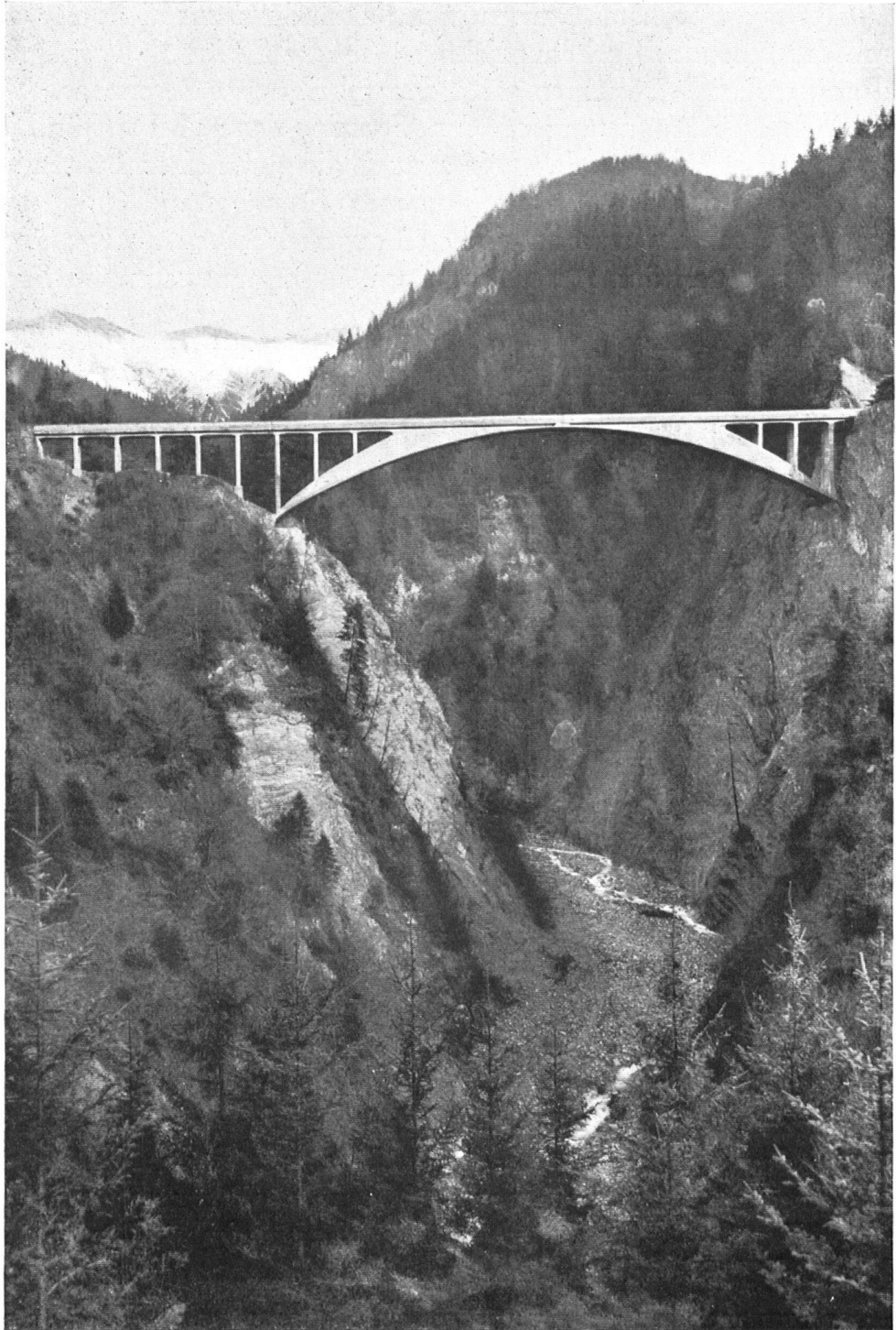
Salginabücke bei Schiers, von Ing. Robert Maillart, Zürich-Genf. Foto: Mischol, Schiers. Pont de la Salgina, près de Schiers (canton des Grisons).
