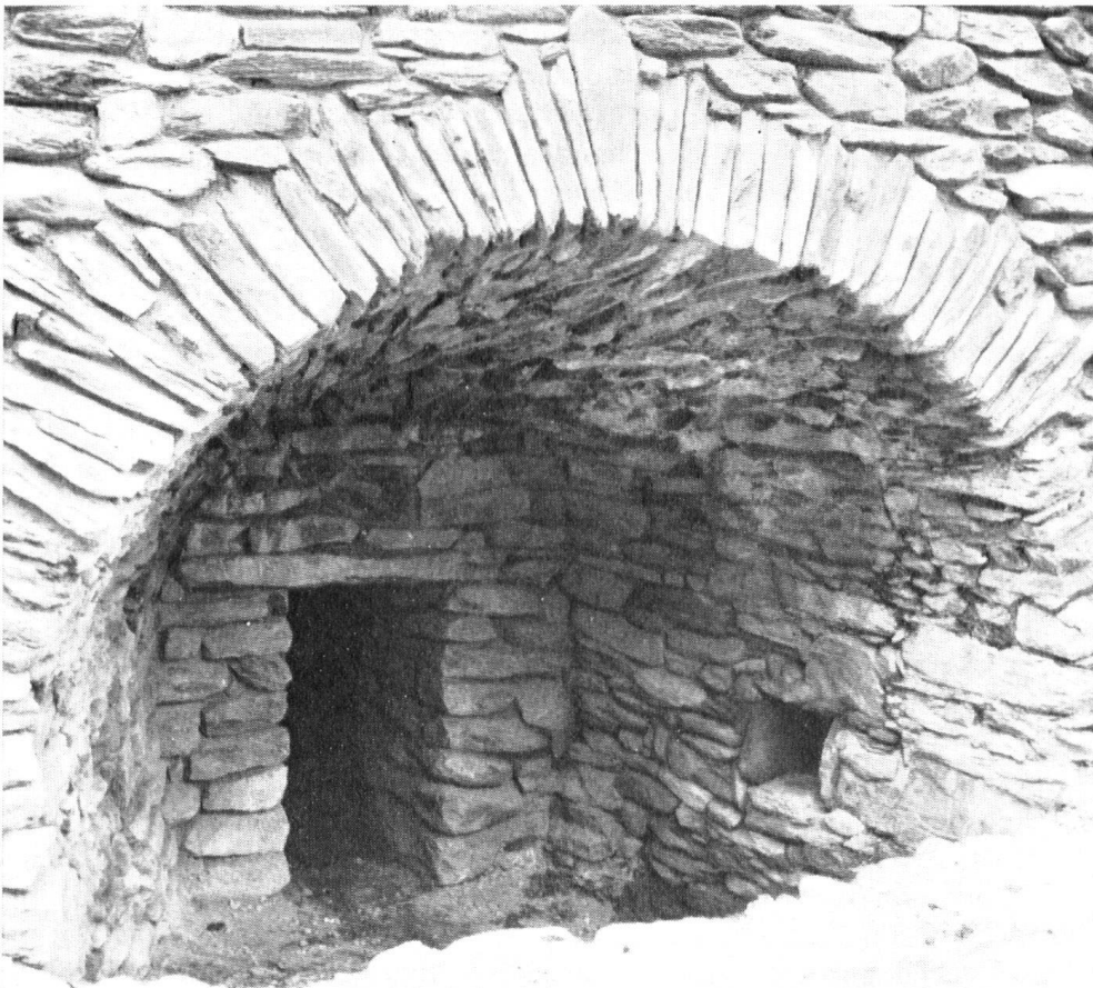
In dieser Form ist der Ofen durch das Restaurationswerk wiedererstand. Die Öffnung bezeichnet die Stelle des einstigen Abstichs; nicht sichtbar (rechts hinten) ist die Formöffnung.
