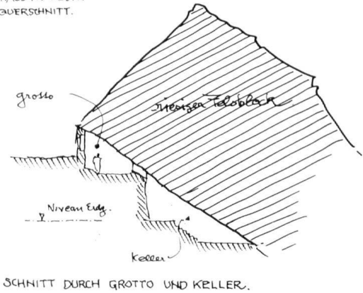
SCHNITT DURCH GROTTO UND KELLER.
