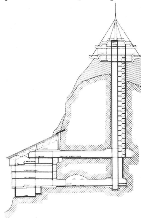
Coupe transversale du projet «Top of Europe», avec son ascenseur conduisant du restaurant à la terrasse panoramique.
