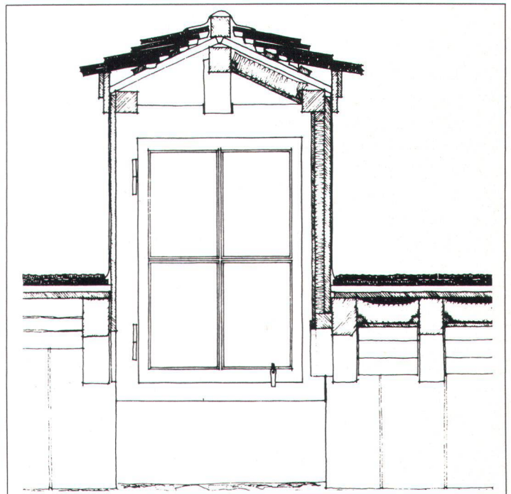
Coupe transversale, vue de l'intérieur: à gauche l'état actuel, à droite un projet d'isolation (illustration Baertschi).
