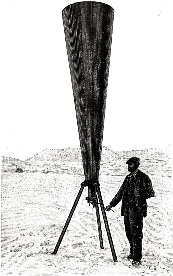
Hagelwetter-Wehrapparat. System Ruef. Hinterlader vermittelt Stahlhülsen.
