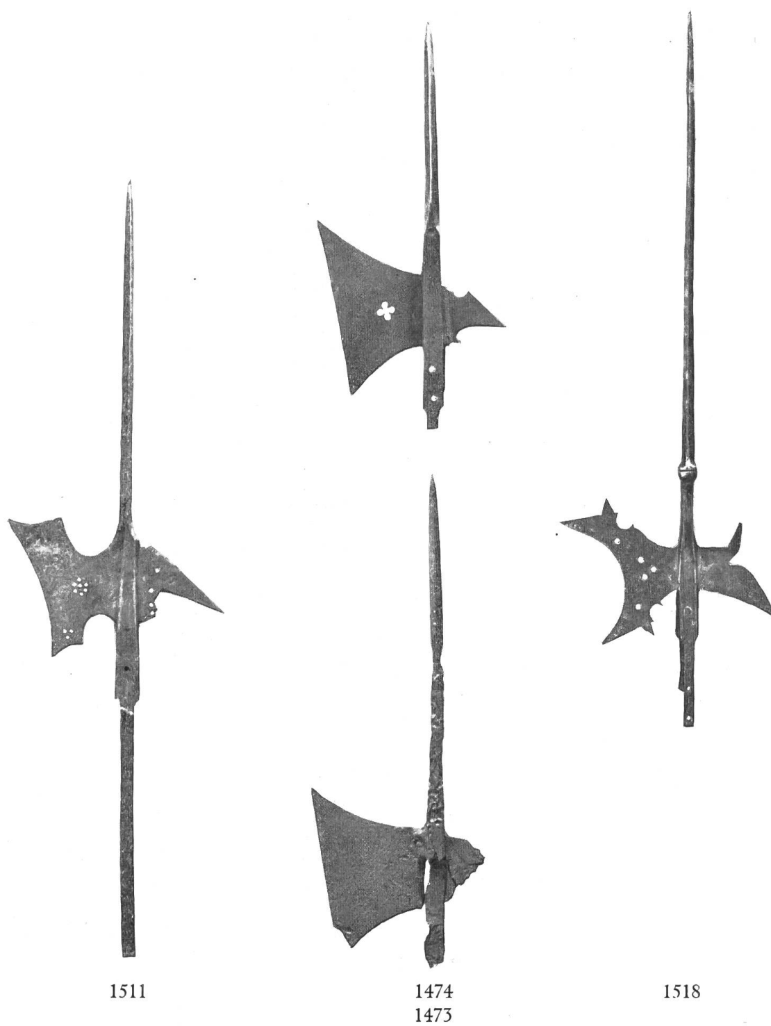
Fig. 45. Halparteneisen. 15.—16. Jahrh.
