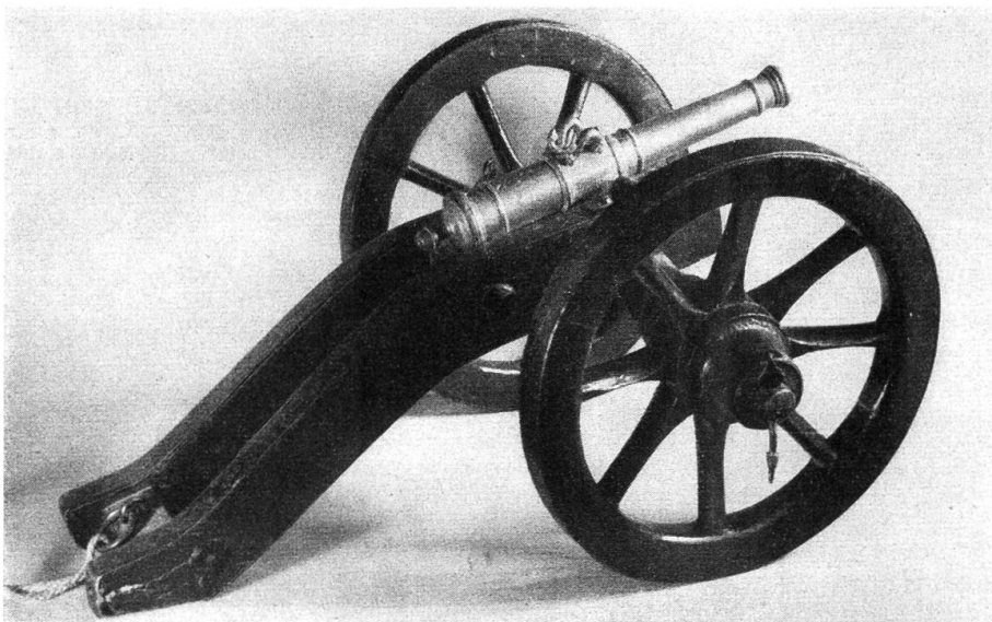
Fig. 171. Knabekanone. 18. Jahrh.
