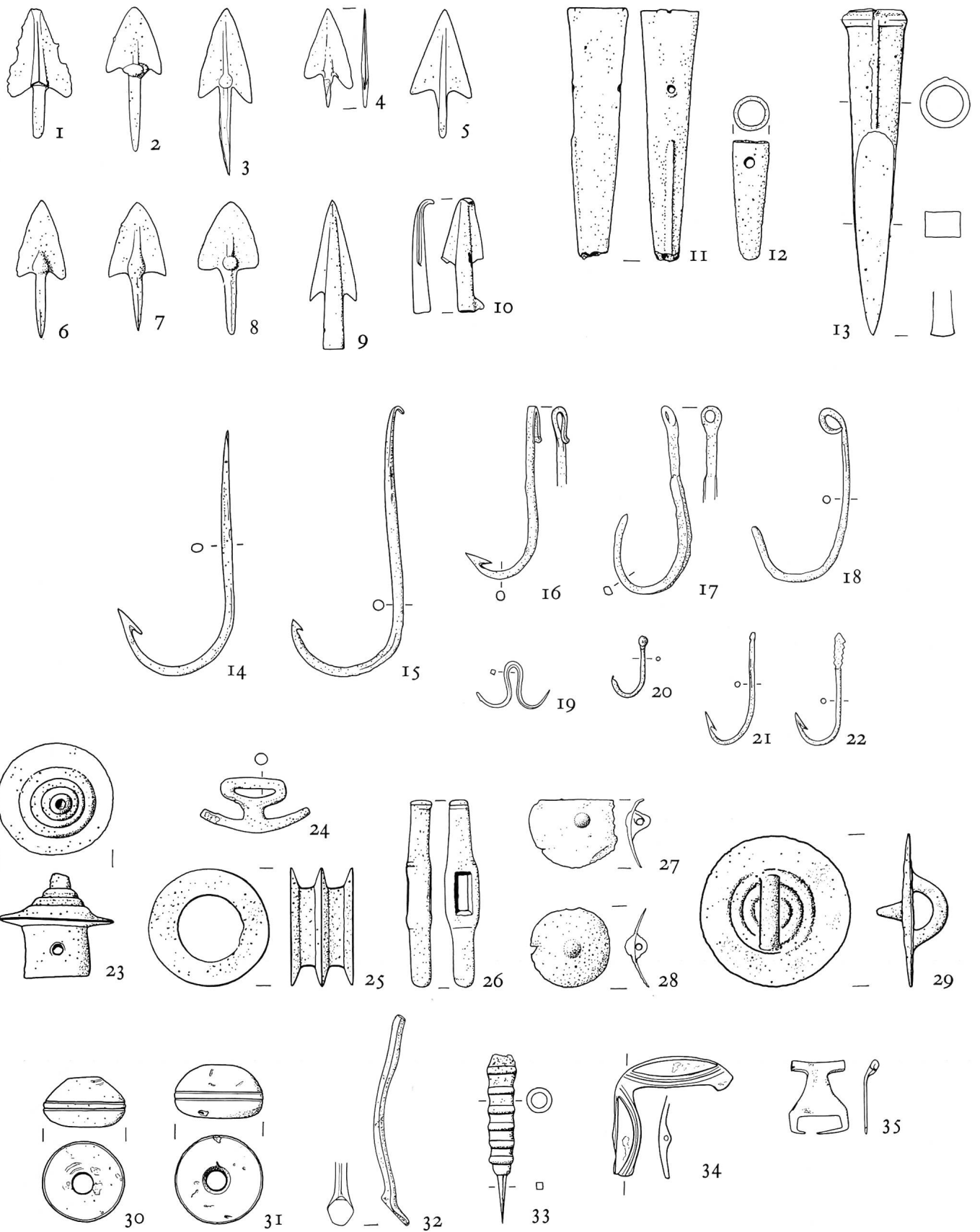
Tafel 13. 1-10 Pfeilspitzen. 11-12 Lanzenschuhe (?). 13 Tüllenmeißel. 14-22 Angelhaken. 23, 25, 32-35 Objekte unbekannter Funktion. 24, 26 Riemenkebel. 27-29 Zierknöpfe. 30-31 Spinnwirtel. 1-29, 32-35 Bronze. 30-31 Ton. M 1 : 2
