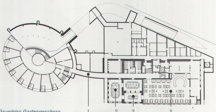
Grundriss Gartengeschoss
