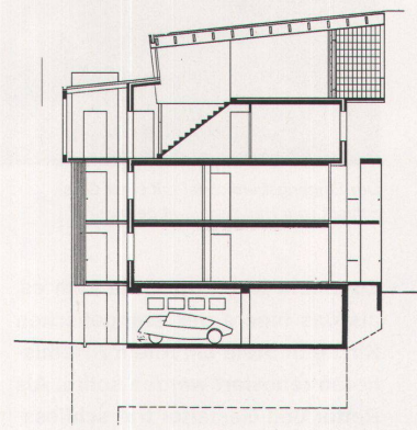
Querschnitt
