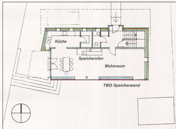
Grundriss Erdgeschoss
