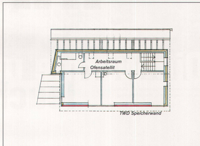
Grundriss Obergeschoss
