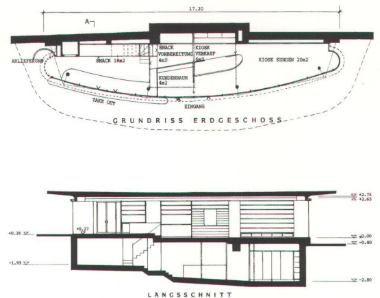
Grundriss des Kiosk und Längsschnitt des Gebäudes mit Unterkellerung
