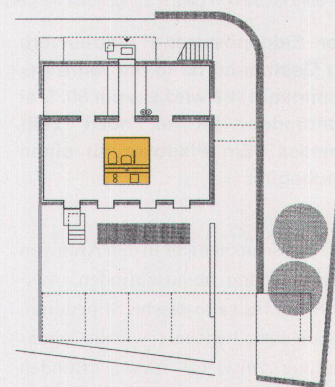
Erdgeschoss des Handwerkerhauses mit Sanitär- und Kücheninsel
