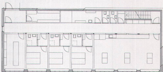
Grundriss Neubau Erdgeschoss
