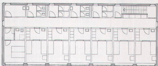
Grundriss Neubau 2. Obergeschoss
