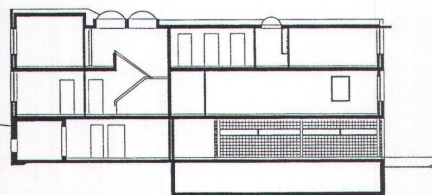
Längsschnitt
