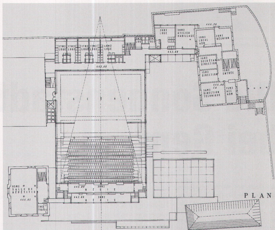
Grundriss auf Bühnenebene
