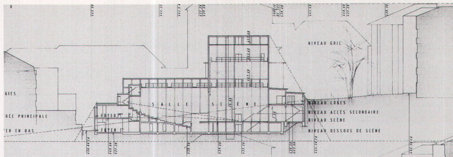
Querschnitt durch Innenraum und Bühne
