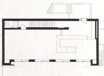
Grundriss Erdgeschoss
