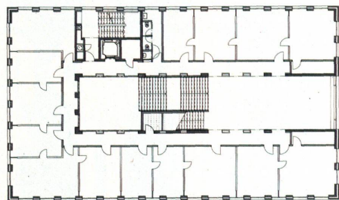
Grundriss 1. OG
