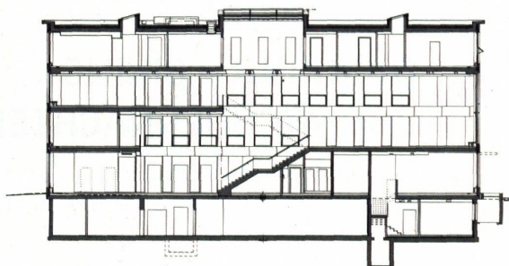
Längsschnitt
