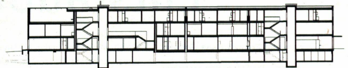
Längsschnitt
