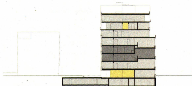
Querschnitt und zwei Grundrisse des Mittelgebäudes: dunkel hervorgehoben eine Splittlevel Wohnung im 2. und 3. Stock
