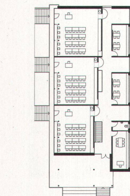
Oben Grundriss Obergeschoss. Rechts das neue Unterrichtsgebäude in Staufen
