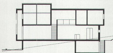
Schnitt
