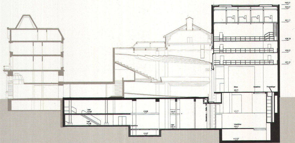
querschnitt mit schwarz eingetragenen umbauten. der bühnenturm wird etwas höher, die raumhöhe im keller grösser. das erlaubt einen effizienteren betrieb. die kellerbühne zieht in den schiffbau um
